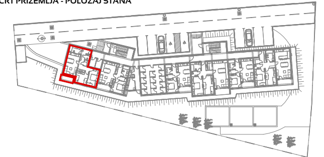
TLOCRT PRIZEMLJA - POLOŽAJ SPREMIŠTA
